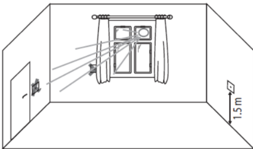
Рис. 5. Рекомендуемые и запрещённые к установке зоны расположения терморегулятора EStemp™ Next Plus.
